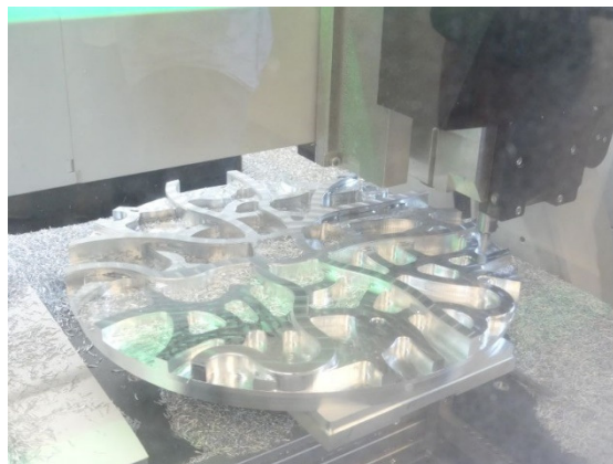
Figure 2 Jante usinée sur DATRON M8Cube, stratégies d'usinage optimisée Mastercam, wheelmaniac.org
